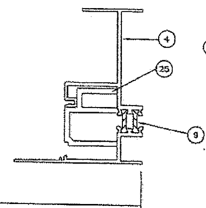
5 JAMB
